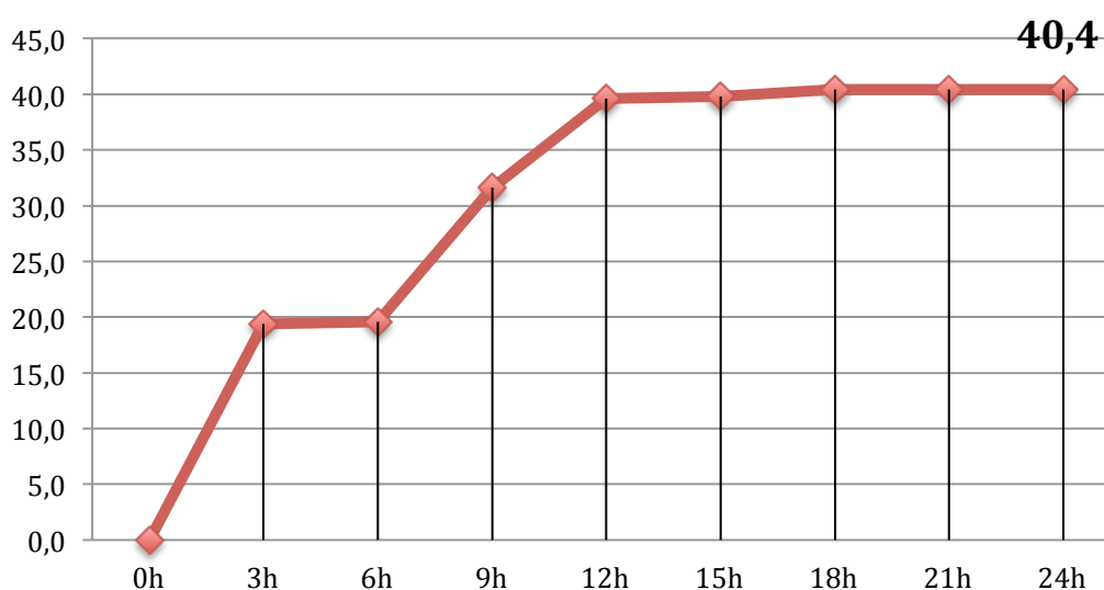
Evolución lluvia acumulada en BARXETA el día 12/09/19 en períodos de 3 horas (en l/m 2 )
