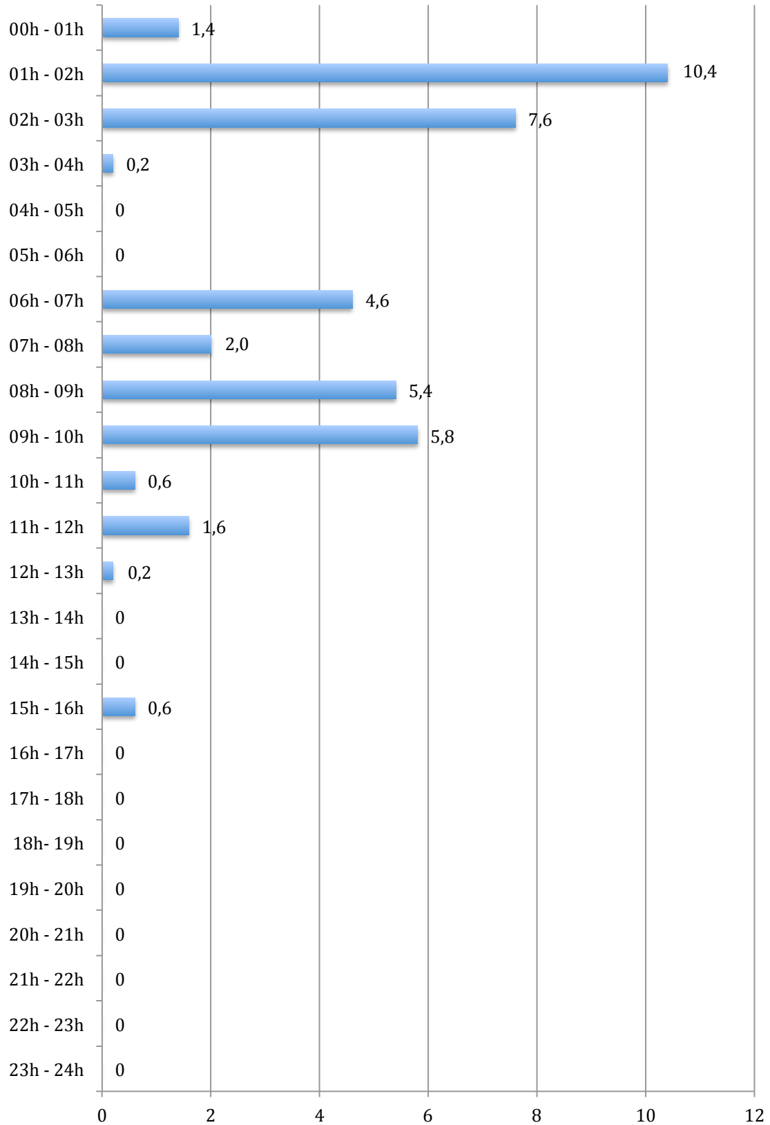
Cantidades de lluvia registradas por horas en BARXETA el día 12/09/19 (en l/m²)
